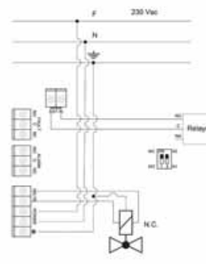
Σχέδιο Σύνδεσης Ηλεκτροβάνας Normally Close
